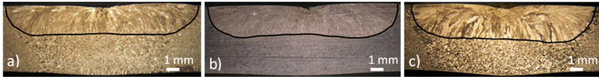
Slika 5.70 Zona taljenja za uzorke s površinom a) u izvornom stanju, b) s brušenom gornjom stranom i c) s brušenom gornjom i donjom stranom; vrijeme zavarivanja 14 s
