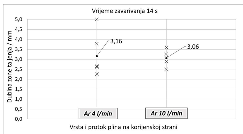
Slika 5.42 Dubine zone taljenja za različite protoke argona na korijenskoj strani zavara
