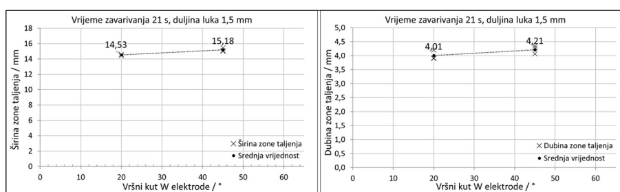
Slika 5.117 Utjecaj vršnog kuta volframove elektrode na širinu i dubinu zone taljenja; duljina električnog luka 1,5 mm
