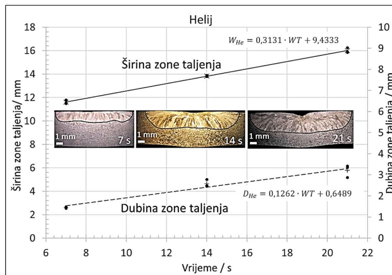
Slika 5.26 Promjena širine i dubine zone taljenja u vremenskom intervalu od 7 s do 21 s, korijenska strana zavara štćena helijem
