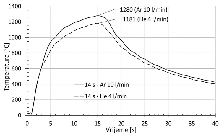
Slika 5.15 Toplinski ciklusi na sredini donje stane uzorka šticiene Ar i He
