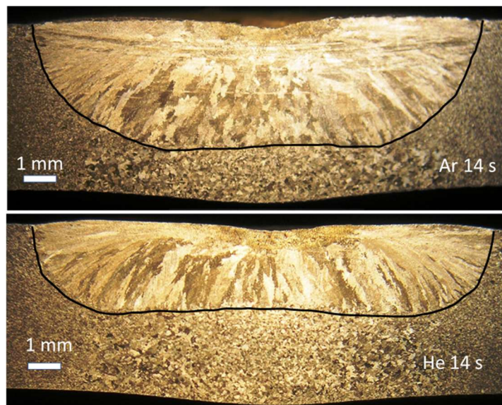
Slika 5.12 Zone taljenja formirane pod zaštitom korijenjske strane zavara Ar i He
