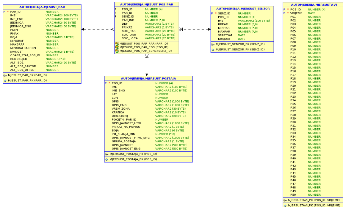
Slika 6.3: Glavne tablice u bazi podataka
