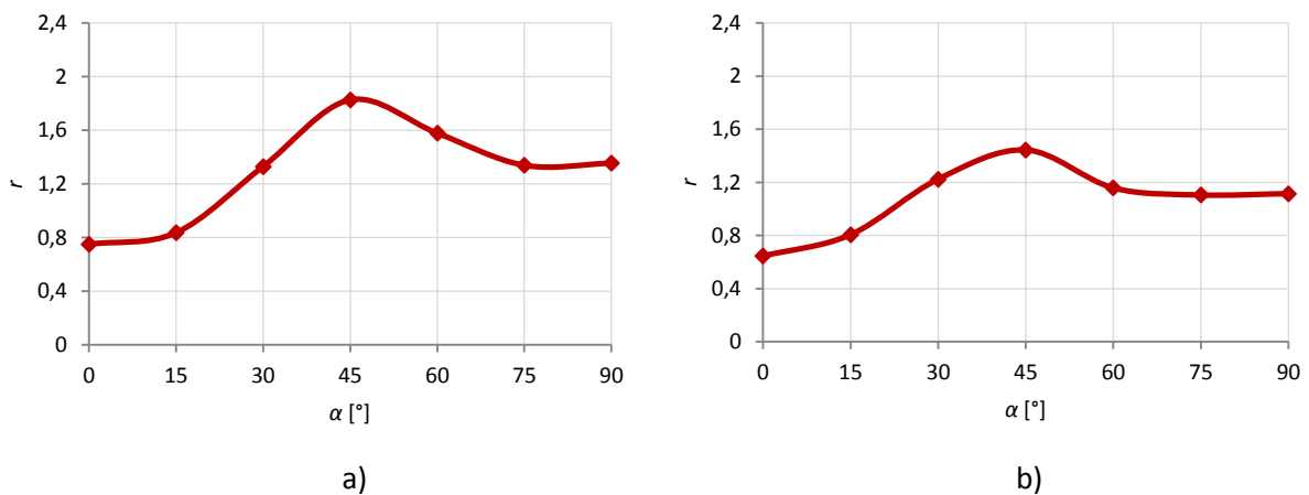
Slika 6.8. Orijeatcijska ovisnost reprezentativnih konstantnih vrijednosti Lankfordovog koeficijenta dobivenih na temelju jednog reprezentativnog uzorka: a) za područje 0 \leq \epsilon^{Np} \leq 0,013 ; b) za područje 0 \leq \epsilon^{Np} \leq 0,006
