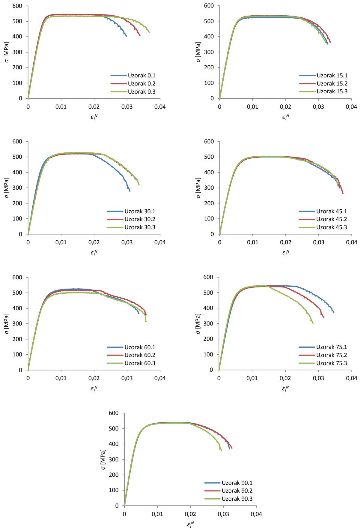
Slika 4.1. Dijagrami ovisnosti stvarnog naprezanja o stvarnoj deformaciji duljine ( \sigma - \epsilon_i^N )
