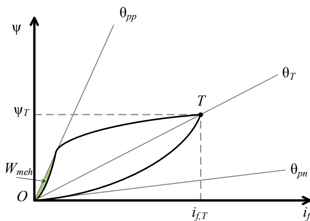
Slika 2.13. Pretvorba magnetske energije u mehaničku
