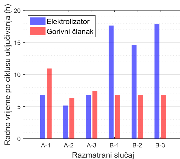
Slika 6.83: Srednje radno vrijeme elektrolizatora i gorivnih članaka po ciklusu uključivanja
