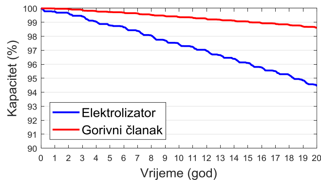
Slika 6.79: Dinamika gubitka kapaciteta elektrolizatora i gorivnog članka, razmatrani slučaj B-3
