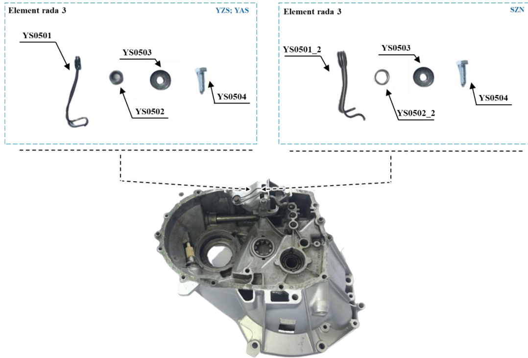
Slika 1.21. Element rada 3
