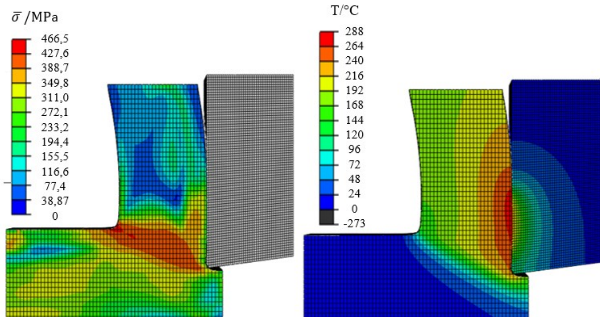
Slika 8.2. Rezultati dobiveni numeričkim postupkom; raspodjela ekvivalentnog naprežanje u obratku i odvojenoj čestici te raspodjela temperature u zoni rezanja za v_c=373 m/min, f = 0,08 mm/o
