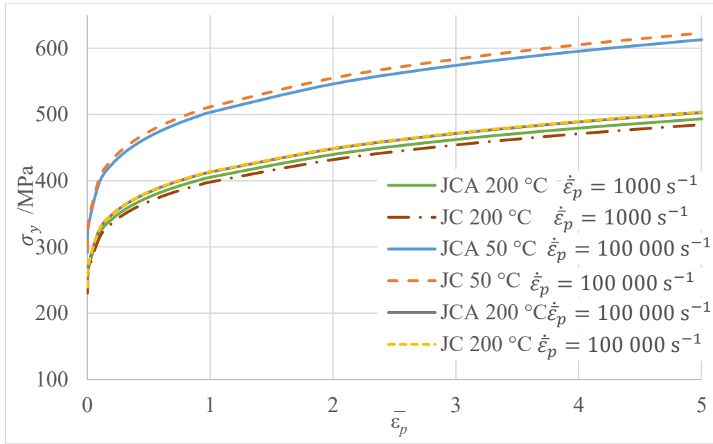
Slika 9.11. Ovisnost naprezanja tečenja o ekvivalentnoj plastičnoj deformaciji za različite zakone očvršćivanja pri razmatranoj vrijednosti \dot{\varepsilon}_p = 1000 \text{ s}^{-1} i \dot{\varepsilon}_p = 100\,000 \text{ s}^{-1}
