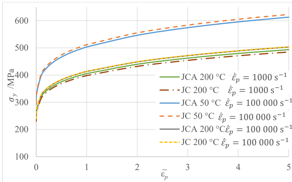
Slika 9.11. Ovisnost naprezanja tečenja o ekvivalentnoj plastičnoj deformaciji za različite zakone očvršćivanja pri razmatranoj vrijednost \dot{\epsilon}_p = 1000 \text{ s}^{-1} i \dot{\epsilon}_p = 100\,000 \text{ s}^{-1}
