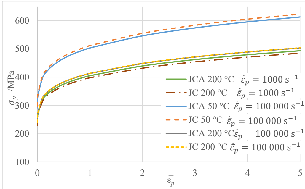
Slika 9.11. Ovisnost naprezanja tečenja o ekvivalentnoj plastičnoj deformaciji za različite zakone očvršćivanja pri razmatranoj vrijednost \dot{\epsilon}_p = 1000 \text{ s}^{-1} i \dot{\epsilon}_p = 100\,000 \text{ s}^{-1}
