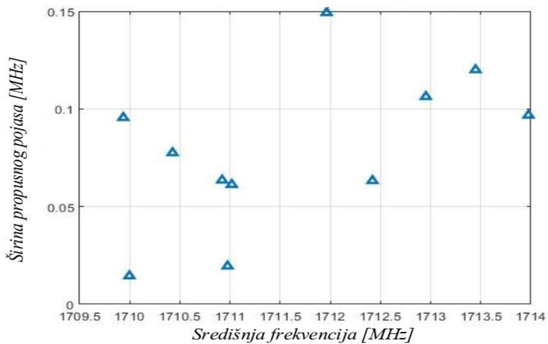
Slika 5.7. Prisutni signali nakon testiranja metode detekcije energije u frekventijskom pojasu od 1710 MHz - 1714 MHz
