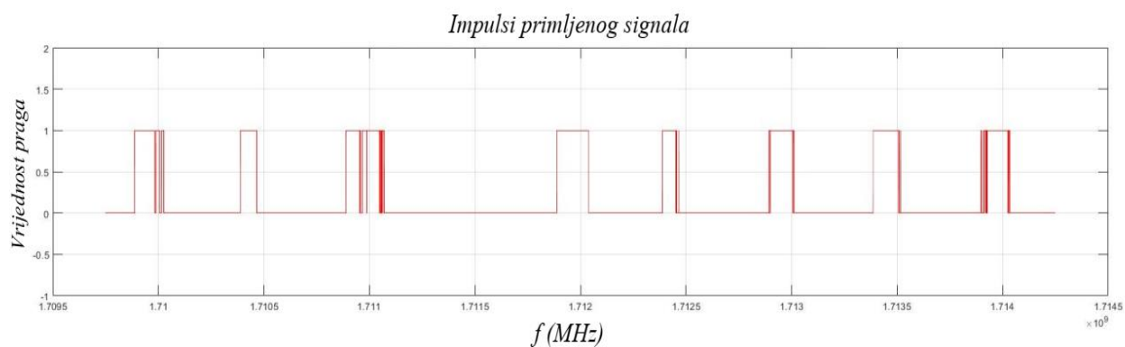
Slika 5.6. Periodogram i impulsi primljenog signala u frekventijskom pojasu od 1710 MHz - 1714 MHz
