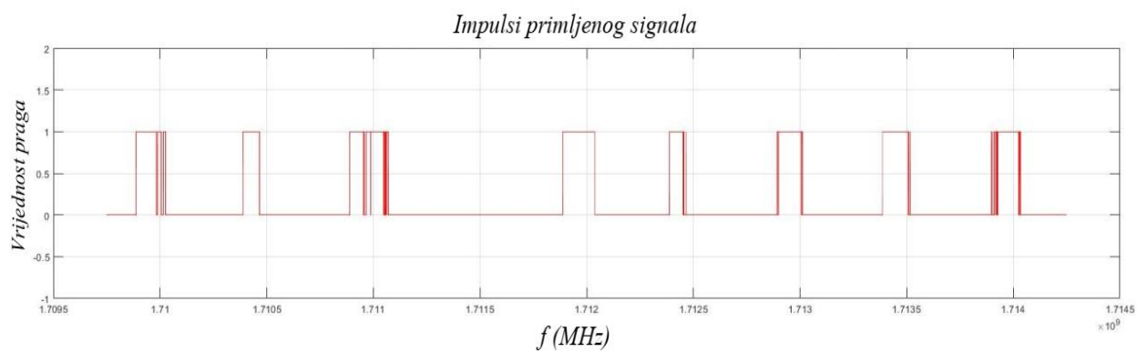
Slika 5.6. Periodogram i impulsi primljenog signala u frekvencijskom pojasu od 1710 MHz - 1714 MHz
