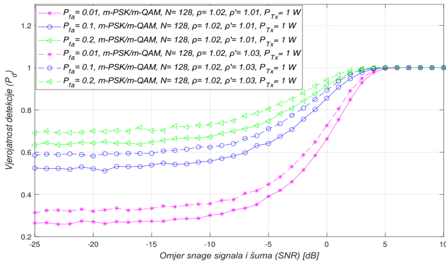
Slika 6.14. Međudnos vjerojatnosti detekcije i omjera snage signala i šuma (SNR-a) za RA sustav s različitim iznosima vjerojatnosti pogrešnog alarma i različitim kombinacijama faktora nesigurnosti snage šuma (NU) i dinamičkog praga detekcije (DDT)
