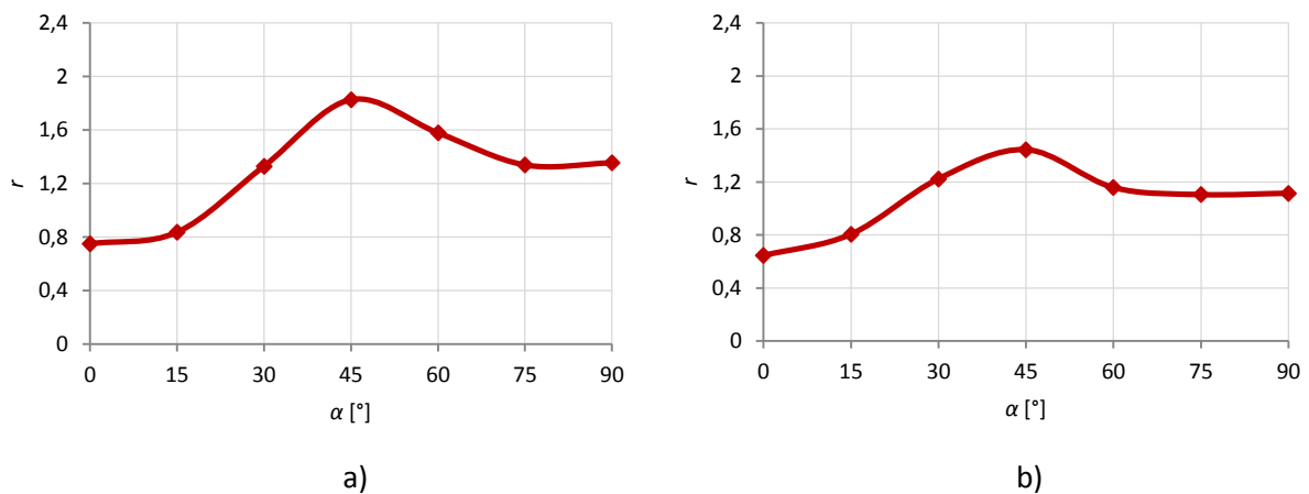
Slika 6.8. Orijehtacijska ovisnost reprezentativnih konstantnih vrijednosti Lankfordovog koeficijenta dobivenih na temelju jednog reprezentativnog uzorka: a) za područje 0 \leq \epsilon^{Np} \leq 0,013 ; b) za područje 0 \leq \epsilon^{Np} \leq 0,006
