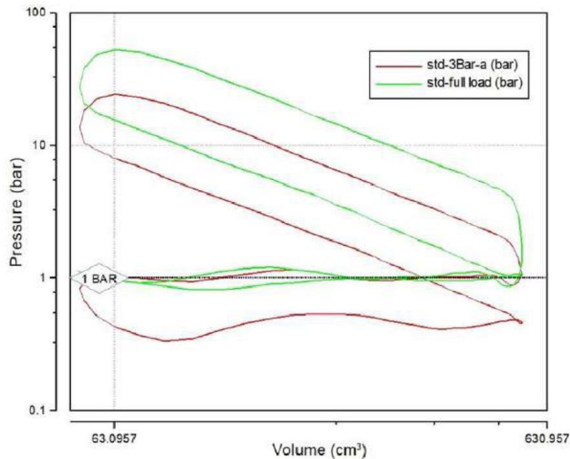
Slika 27. Indicatorski dijagrami testiranog motora [1].
