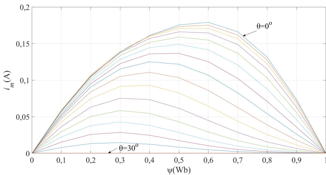
Slika 4.14. Ovisnost struje kroz nadomjesni otpor gubitaka u željezu o položaju i magnetskom toku
