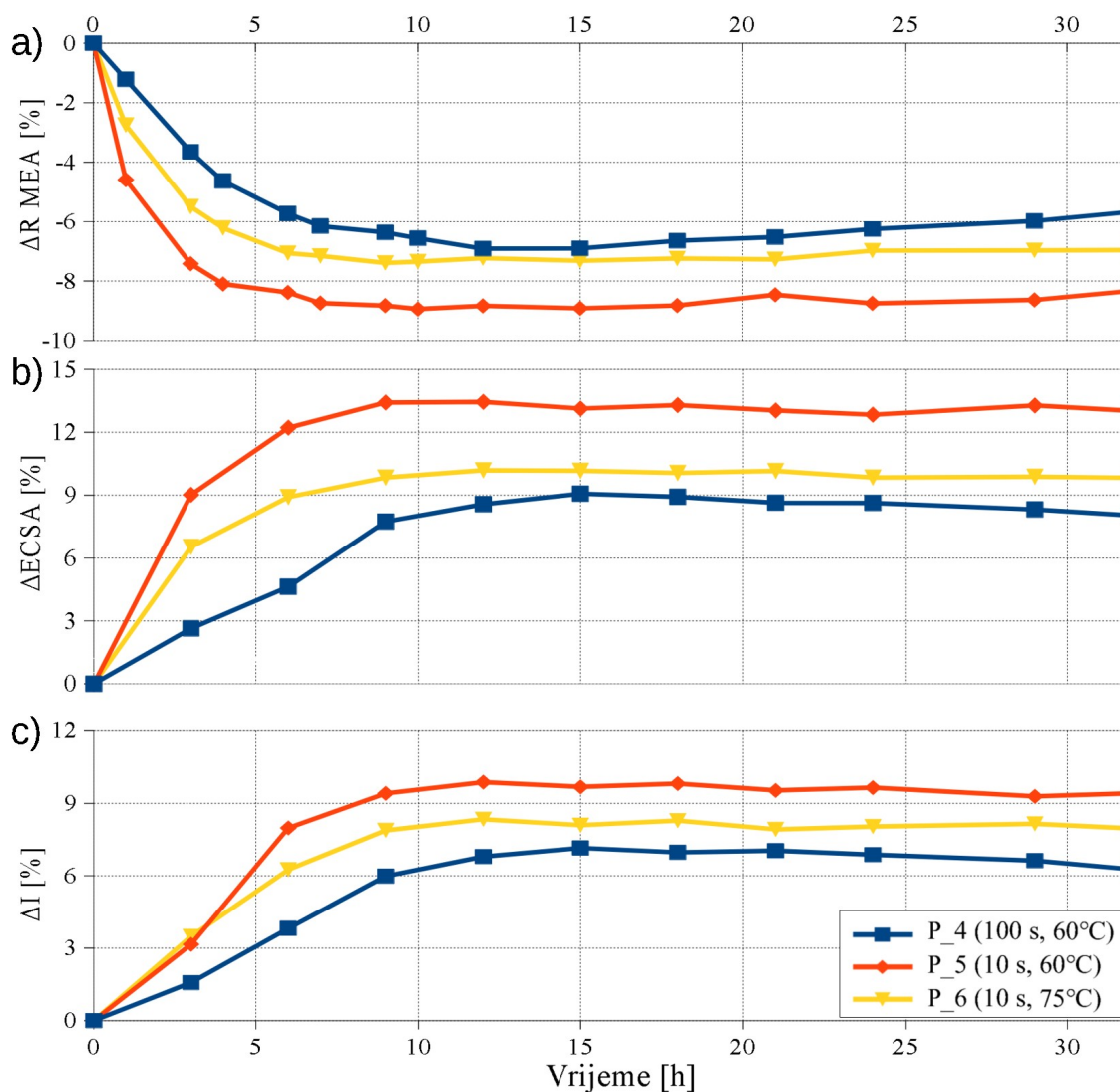
Slika 5.13. Promjene mjenjenih veličina tijekom aktivacijskih postupaka pri cikliranju radne točke 2. faze istraživanja, otpor membrane a), elektrokemijska aktivna površina b), maksimalna struja c)
