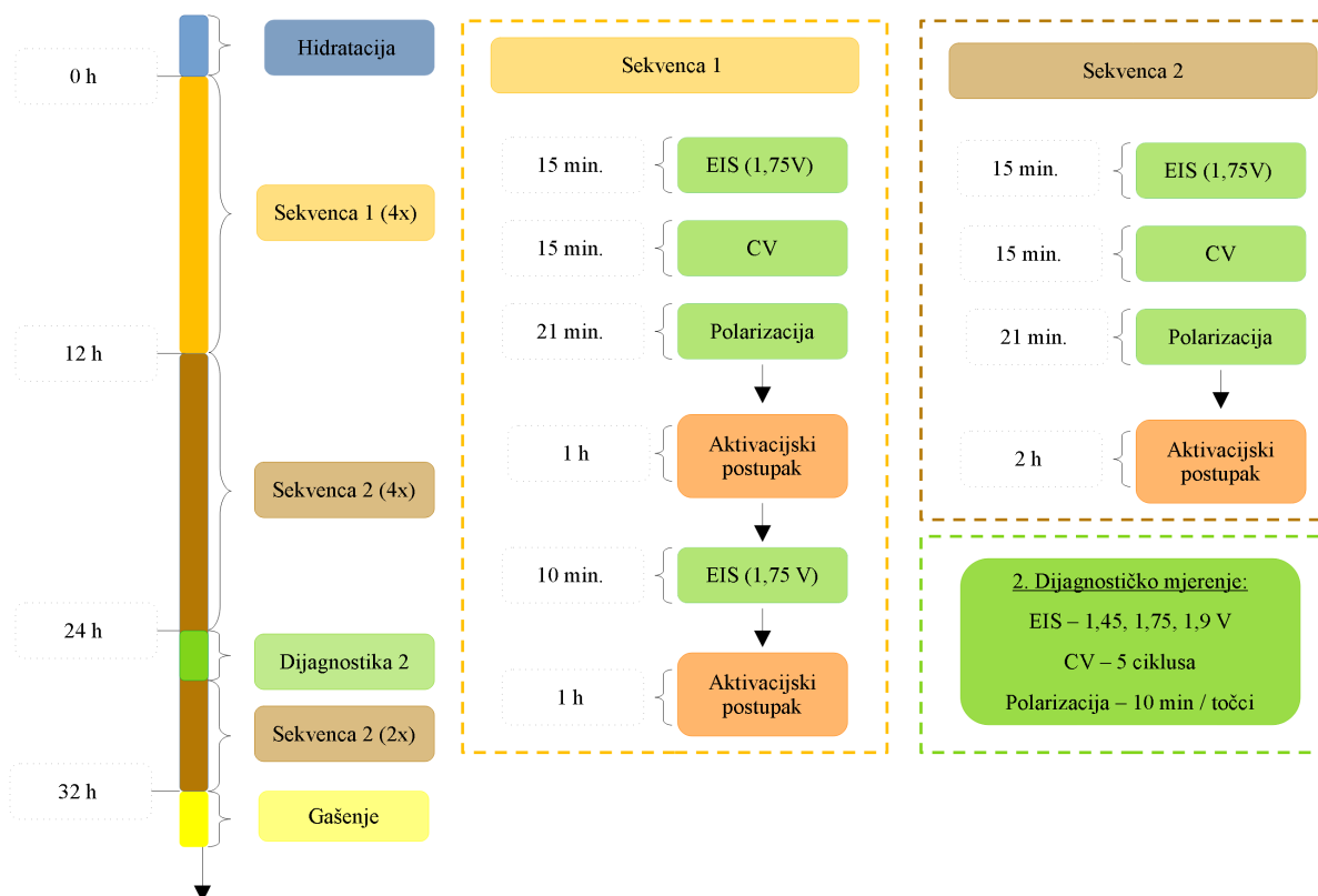
Slika 4.2. Protokol za praćenje aktivacijskog postupka 2. faze istraživanja
