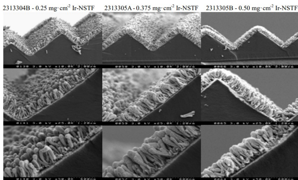
Slika 2.4. SEM slike nanostrukturiranog Ir-NSTF “whiskers” potpornog sloja [18]
