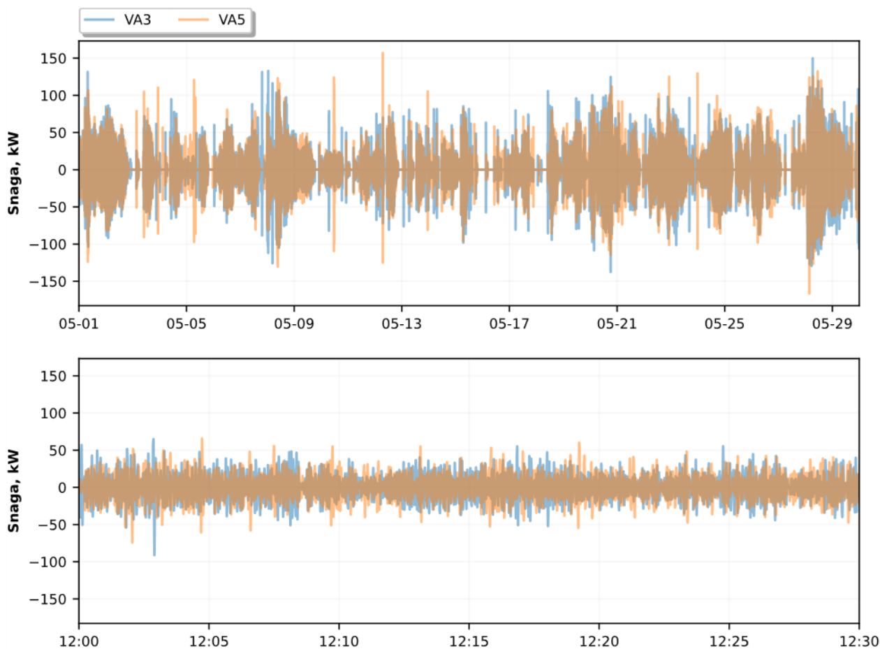
Slika 5-26 Usporedba drugog detaljnog koeficijent (D2) MODWT MRA za dva različita VA u VE
