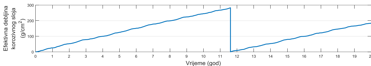
Slika 6.77: Dinamika prirasta efektivnog korozivnog sloja, razmatrani slučaj B-3
