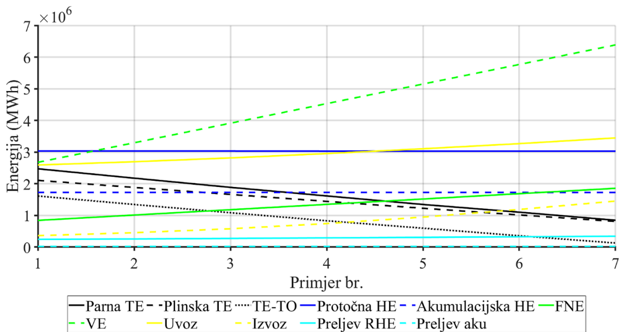
Slika 3.42 Energije ostalih proizvođača u slučaju povećanja proizvodnje IOIE
