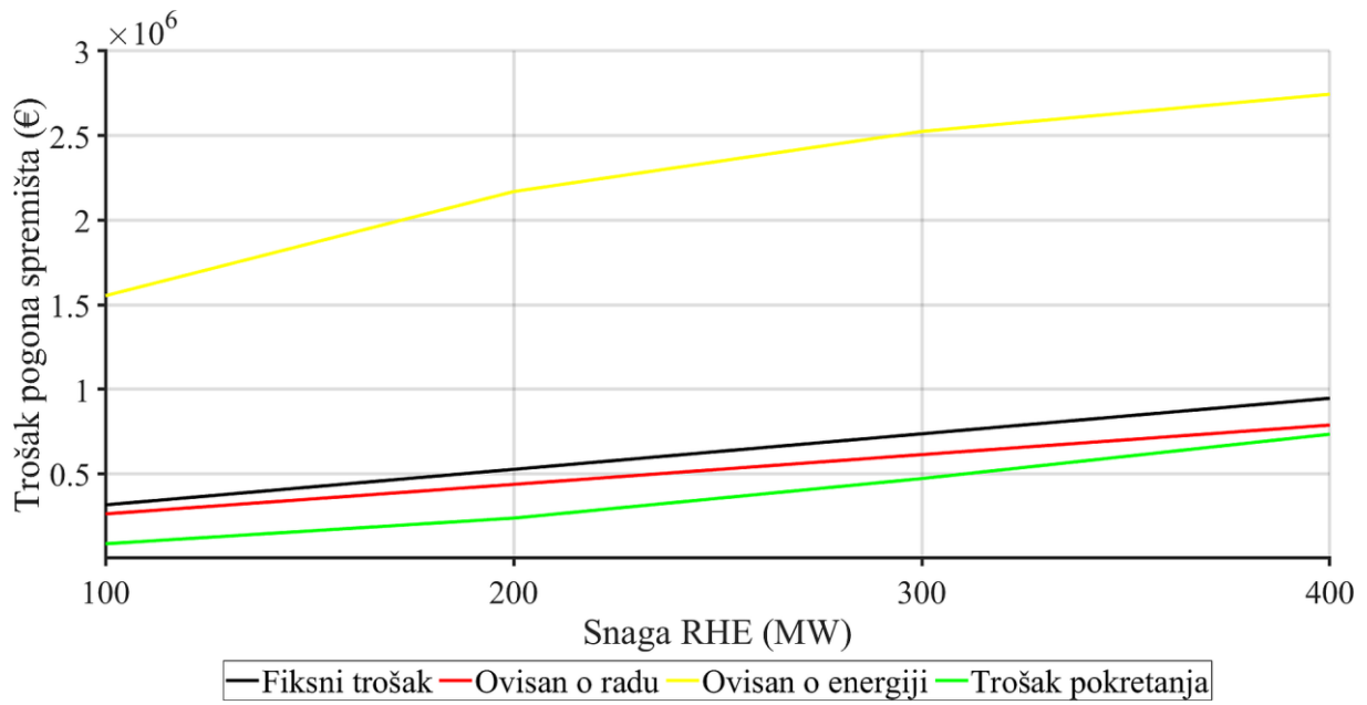
Slika 3.23 Troškovi pogona RHE u slučaju GENCO-a
