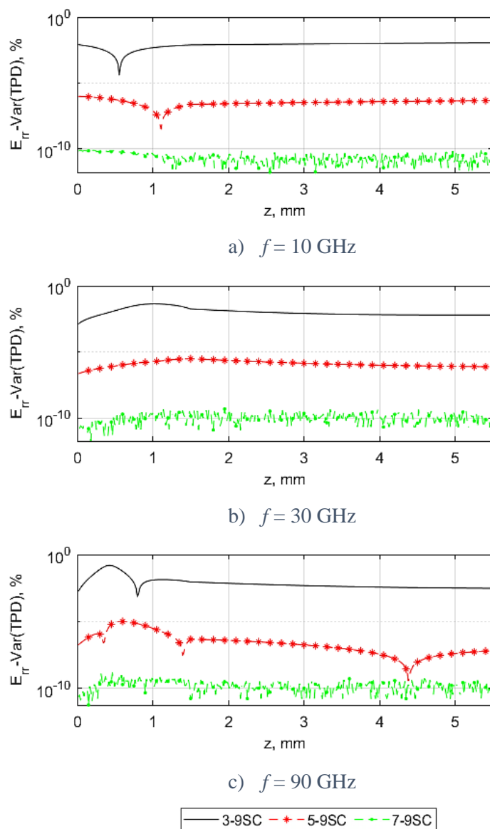
Slika 8.53 Konvergencija SC metode pri izračunu varijanci TPD. Referentna razina dobivena je iz varijance s 9 kolokacijskih točaka
