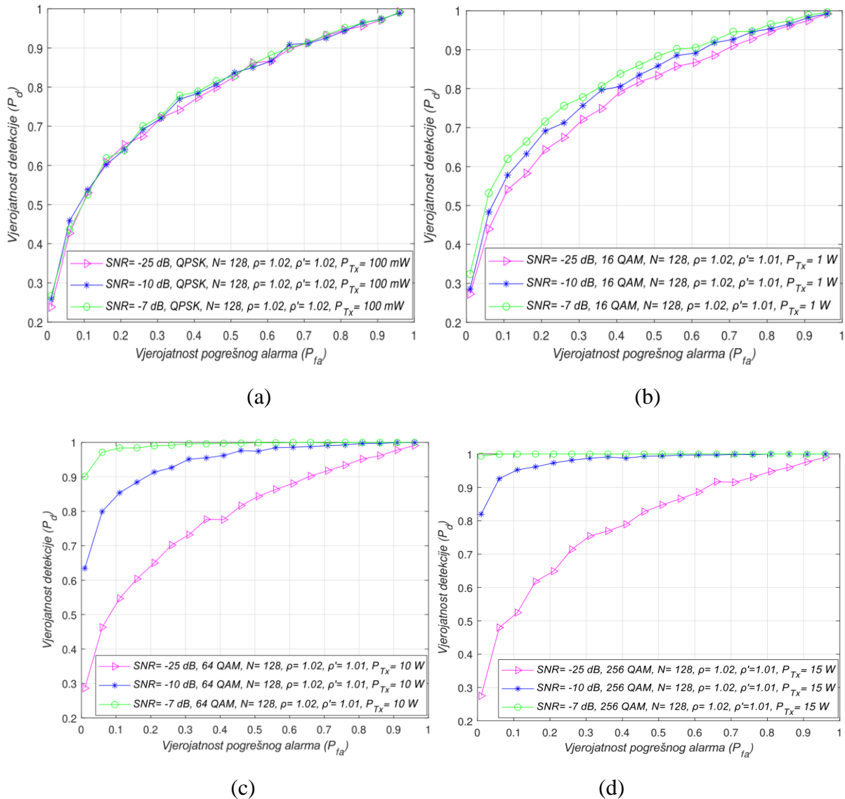
Slika 6.9. Krivulje radnih karakteristika prijemnika (ROC krivulje) za proces detekcije energije (ED) m-PSK/m-QAM moduliranih signala s različitim razinama omjera snage signala i šuma (SNR-a) kada se signal primarnog korisnika (PU) odašilje s: (a) 0,1 W; (b) 1 W; (c) 10 W i (d) 15 W
