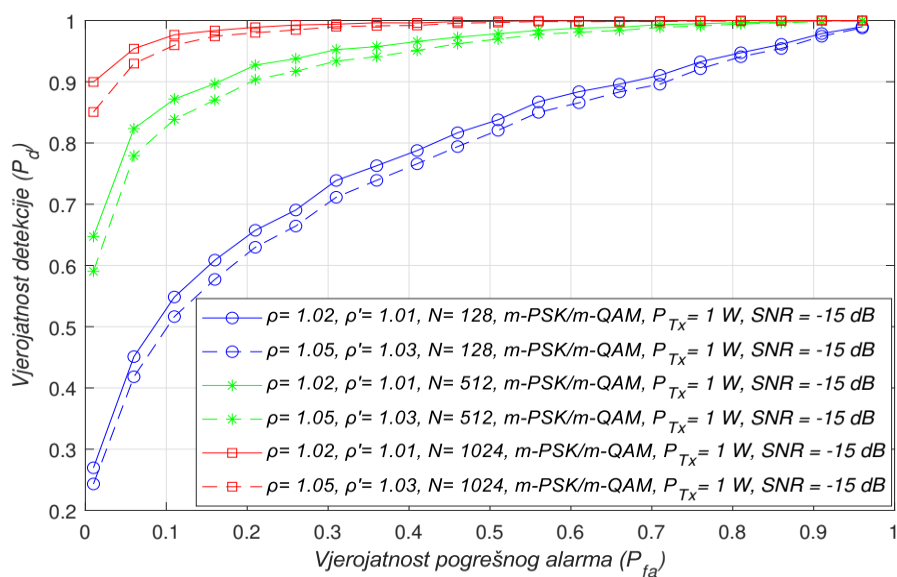
Slika 6.11. Krivulje radnih karakteristika prijemnika (ROC krivulje) procesa detekcije energije (ED) za m -PSK/ m -QAM signale odašlane sa snagom odašiljanja ( P_{Tx} ) od 1 W i detektiranih s različitim količinama uzoraka
