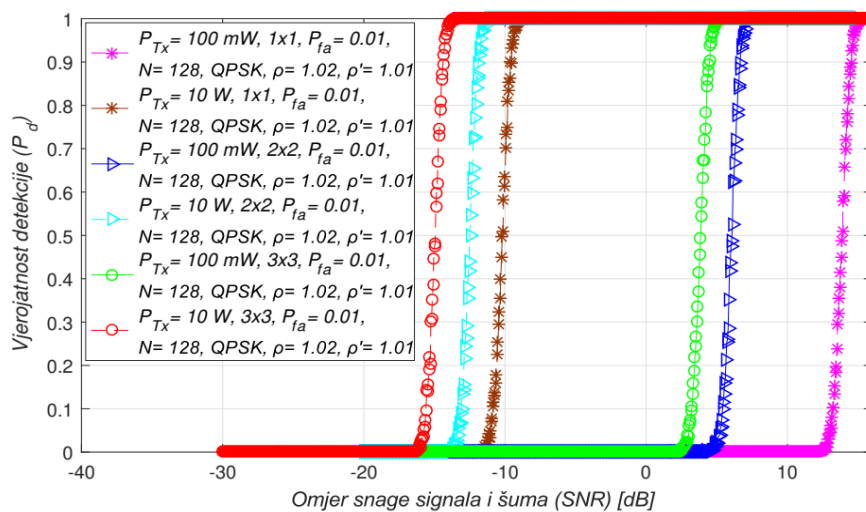
Slika 7.11. Međuviznost vjerojatnosti detekcije i omjera snage signala i šuma (SNR-a) u procesu detekcije energije (ED) signala koji se prenose s različitim snagama odašiljanja (Tx) primarnog korisnika (PU) u simetričnim MIMO sustavima prijenosa
