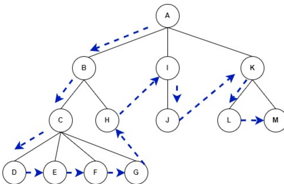
Slika 2.6. Ilustracija pretraživanja po dubini
