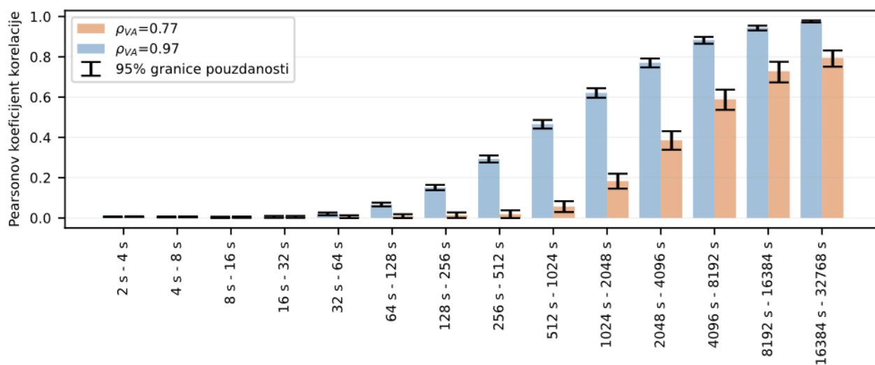
Slika 5-10 Koeficijent korelacije različitih vremenskih skala između dva VA na lokaciji „A“ i „C“
