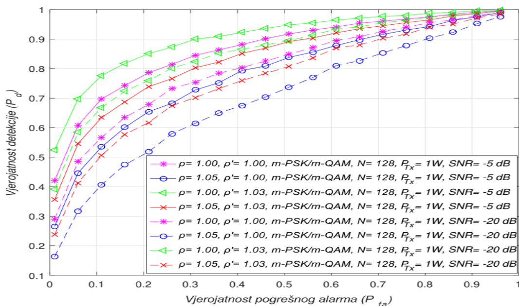
Slika 6.4. Krivulje radnih karakteristika prijelnika (ROC krivulje) za signale u RA sustavima s različitim kombinacijama faktora nesigurnosti snage šuma ( NU ) i dinamičkog praga detekcije (DDT) i dvije različite razine omjera snage signala i šuma (SNR)
