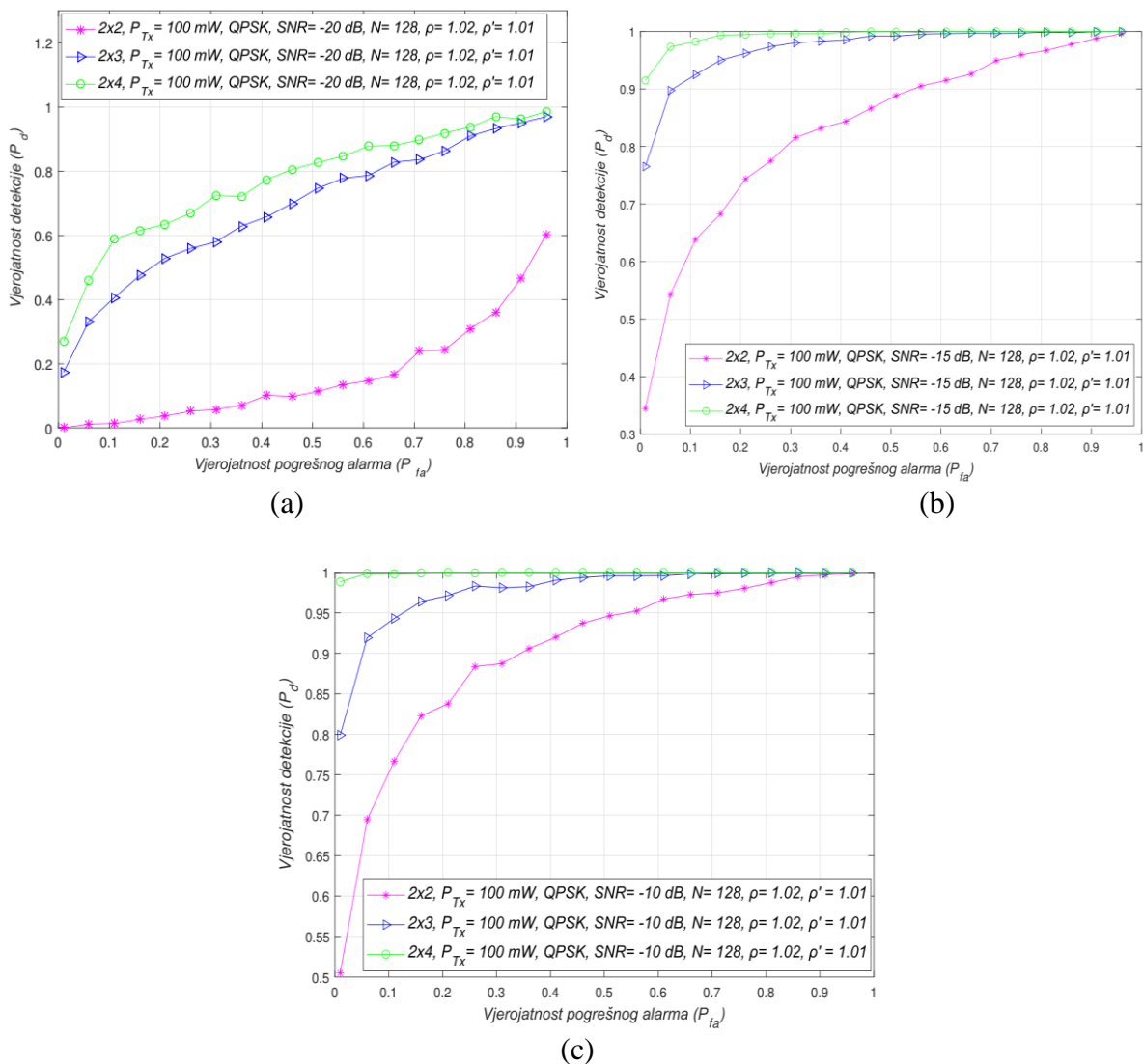
Slika 7.19. Krivulje radnih karakteristika prijemnika (ROC krivulje) analizirane metode detekcije energije (ED) za različite vrijednosti omjera snage signala i šuma (SNR-a) jednake: (a) -20 dB, (b) -15 dB i (c) -10 dB
